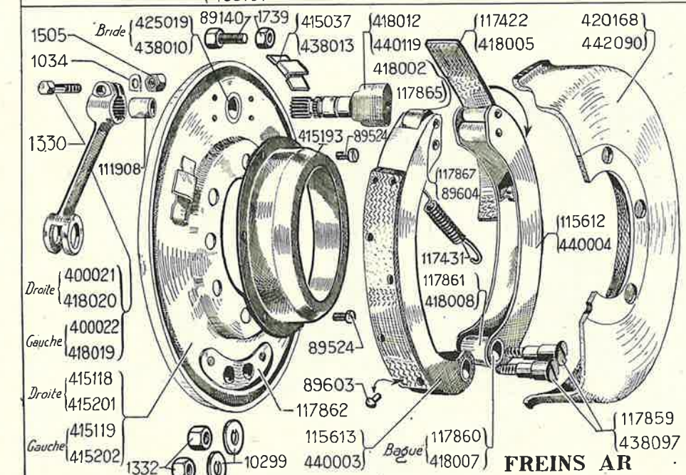
FREINS AV
